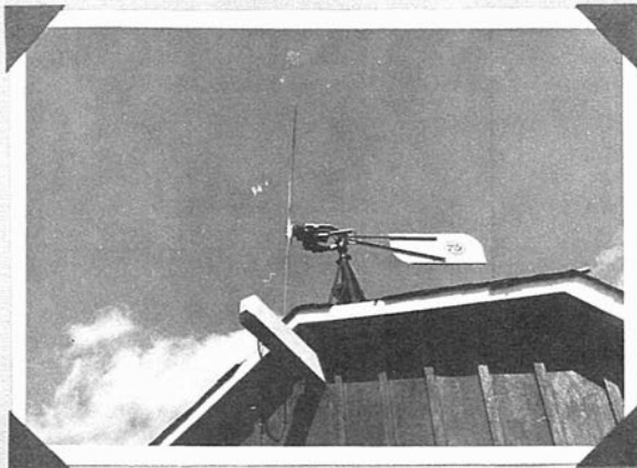
PHOTO 8. Deleo 200 Watt - 12 Volt
